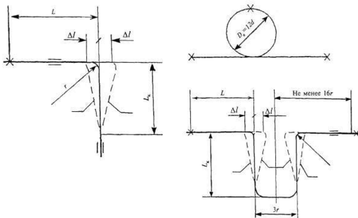
Рисунок Д.1. - Расчетные схемы гнутых компенсаторов
